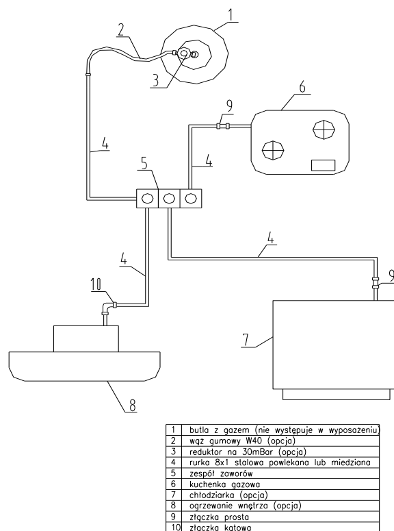
Rys.8. Schemat instalacji gazowej.
